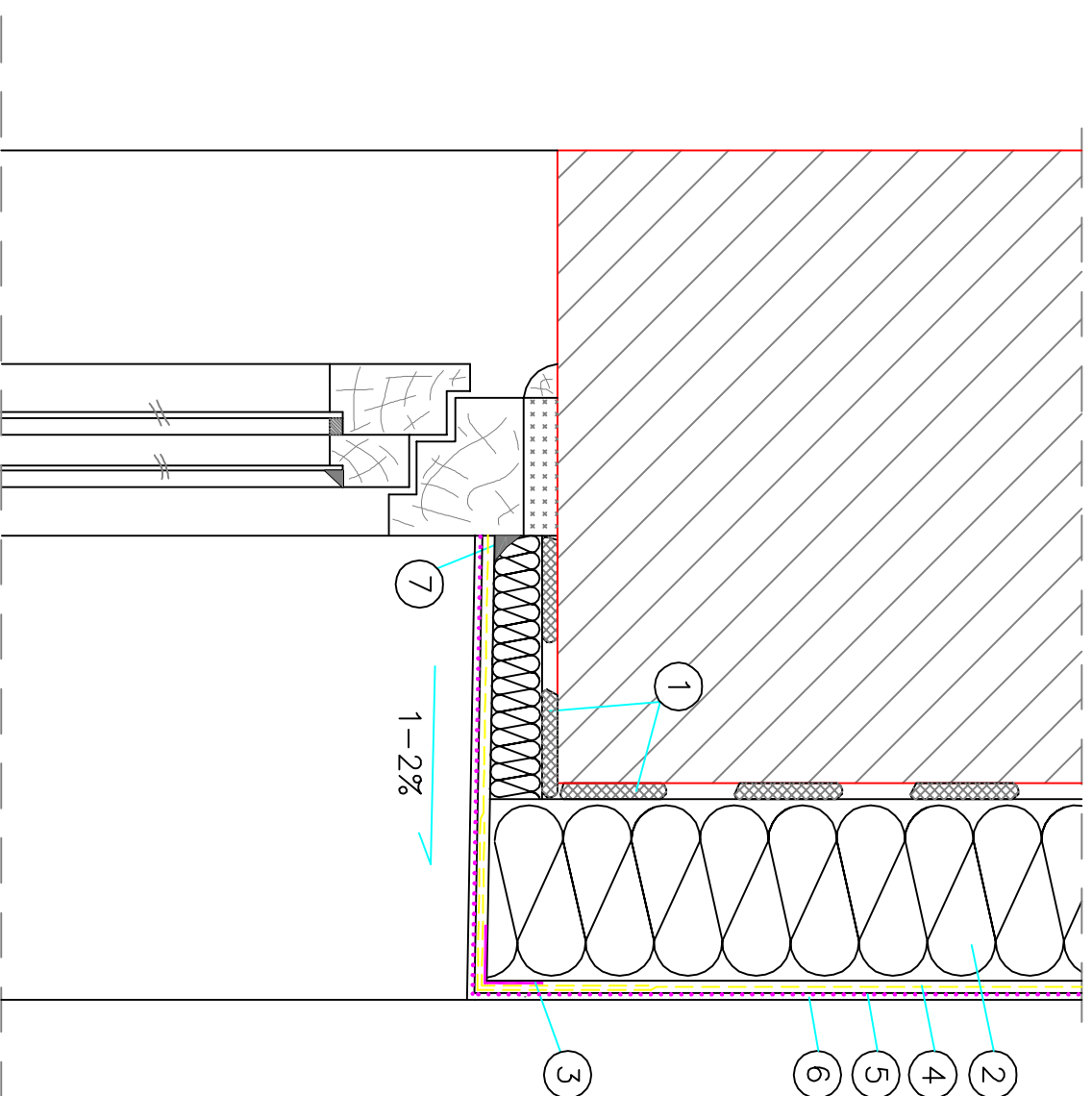
Rys. 7.16 Docieplenie nadproża
