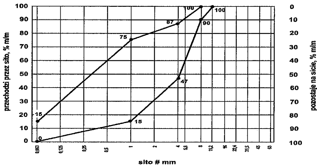
Rys. 1. Krzywe graniczne uziarnienia mieszanki kruszywa 0/8 mm do górnej warstwy podłoża ulepszanego
