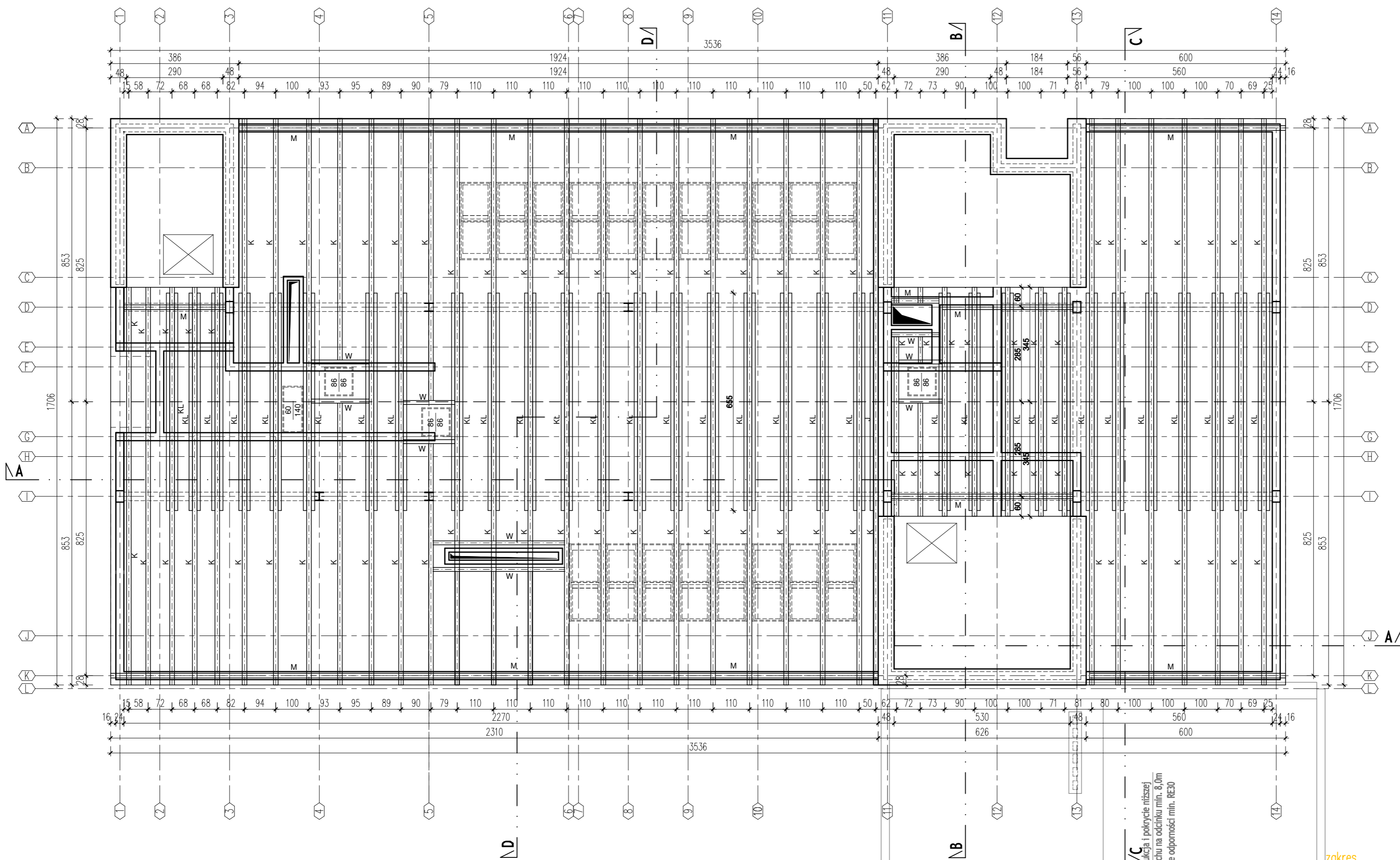
RZUT WIĘZBY DACHOWEJ
