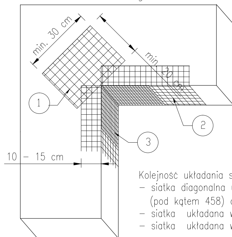
Szczegół A
