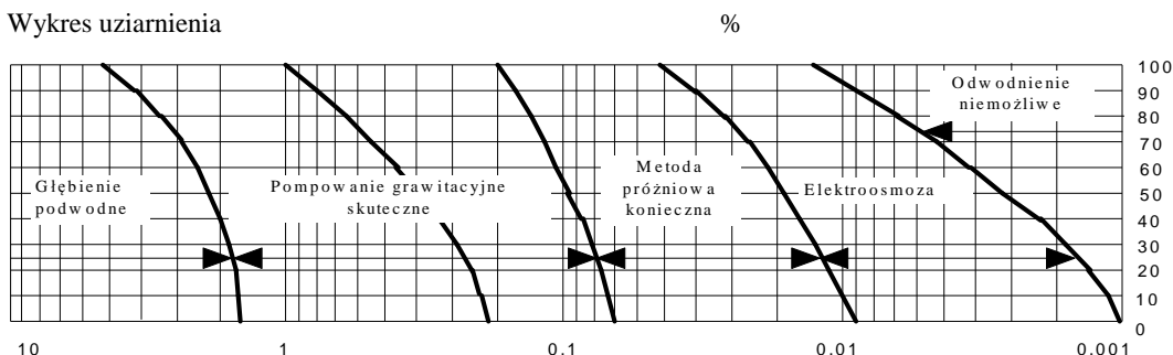
Wykres uziarnienia
