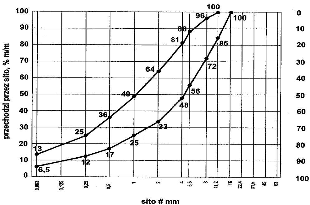
Rys. 4. Krzywe graniczne uziarnienia mieszanki mineralnej 0/11,2 mm
