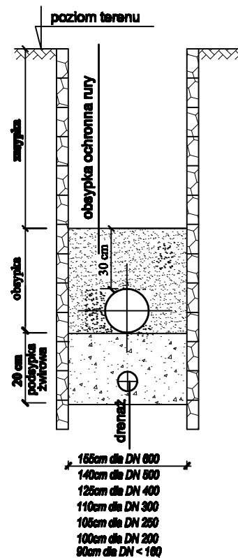
Wykop szalowany - woda gruntowa odwodnienie drenażem
