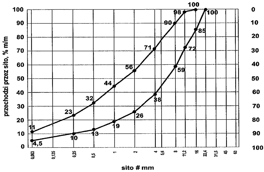
Rys. 3. Krzywe graniczne uziarnienia mieszanki mineralnej 0/16 mm
