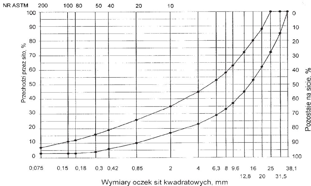
Rys.1. Krzywe graniczne uziarnienia mieszanki mineralnej BA od 0 do 31,5 mm do podbudowy nawierzchni drogi o obciążeniu ruchem KR 1 lub KR 2
