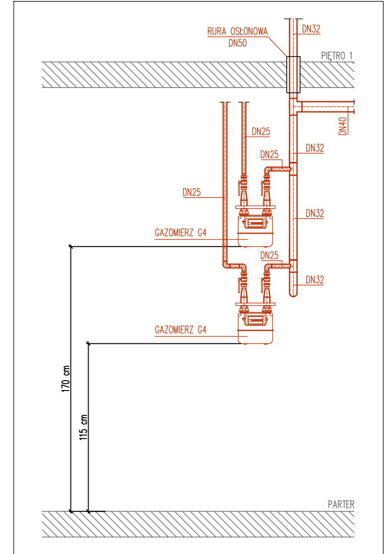
SCHEMAT A – PODŁĄCZENIE GAZOMIERZY NA PARTERZE
