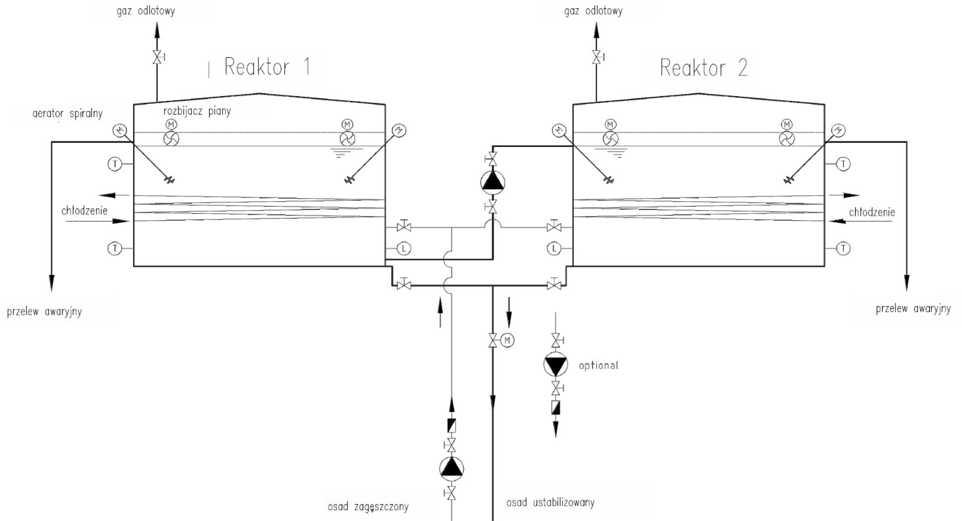
Rysunek 2. Schemat technologiczny procesu ATSO
