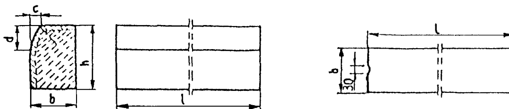
Rys. 1. Wymiarowanie krawężników
